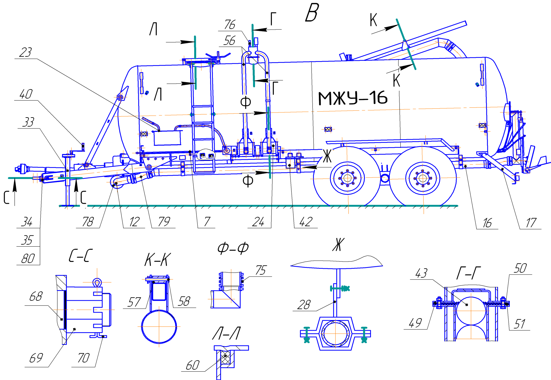
Рисунок 1.3 – Машина МЖУ-16
