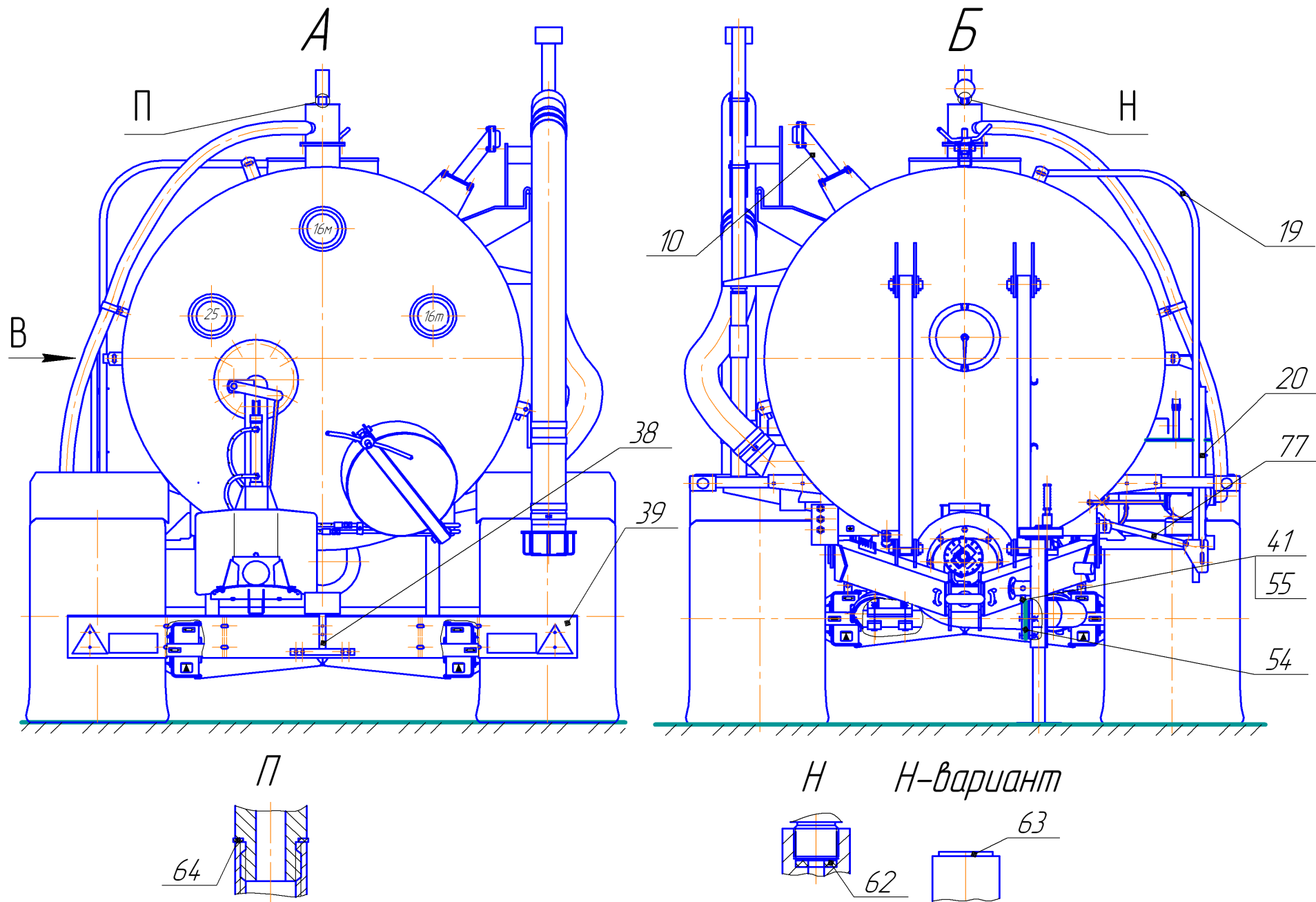
Рисунок 1.2 – Машина МЖУ-16
