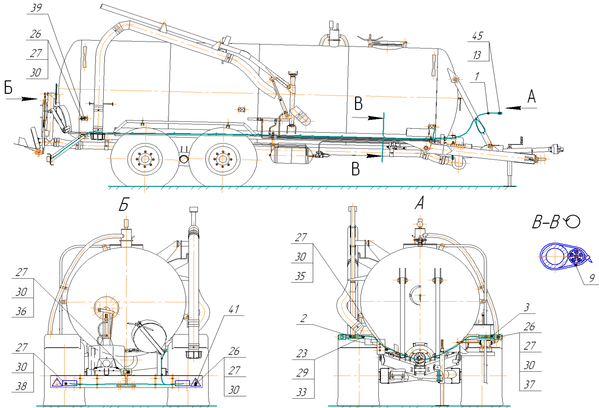
Рисунок 3 – Электрооборудование МЖУ-16.27.00.000
