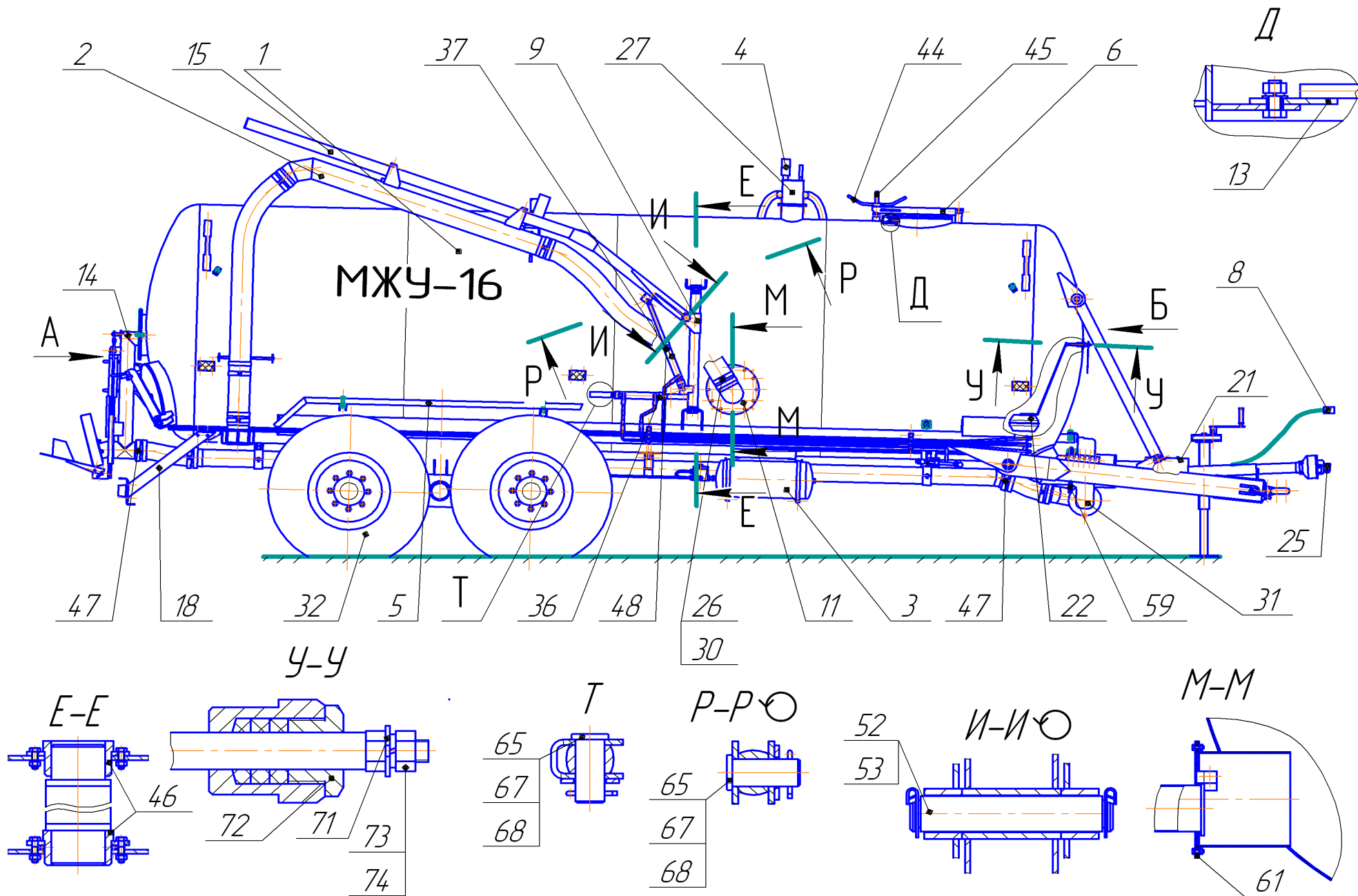
Рисунок 1.1 – Машина МЖУ-16
