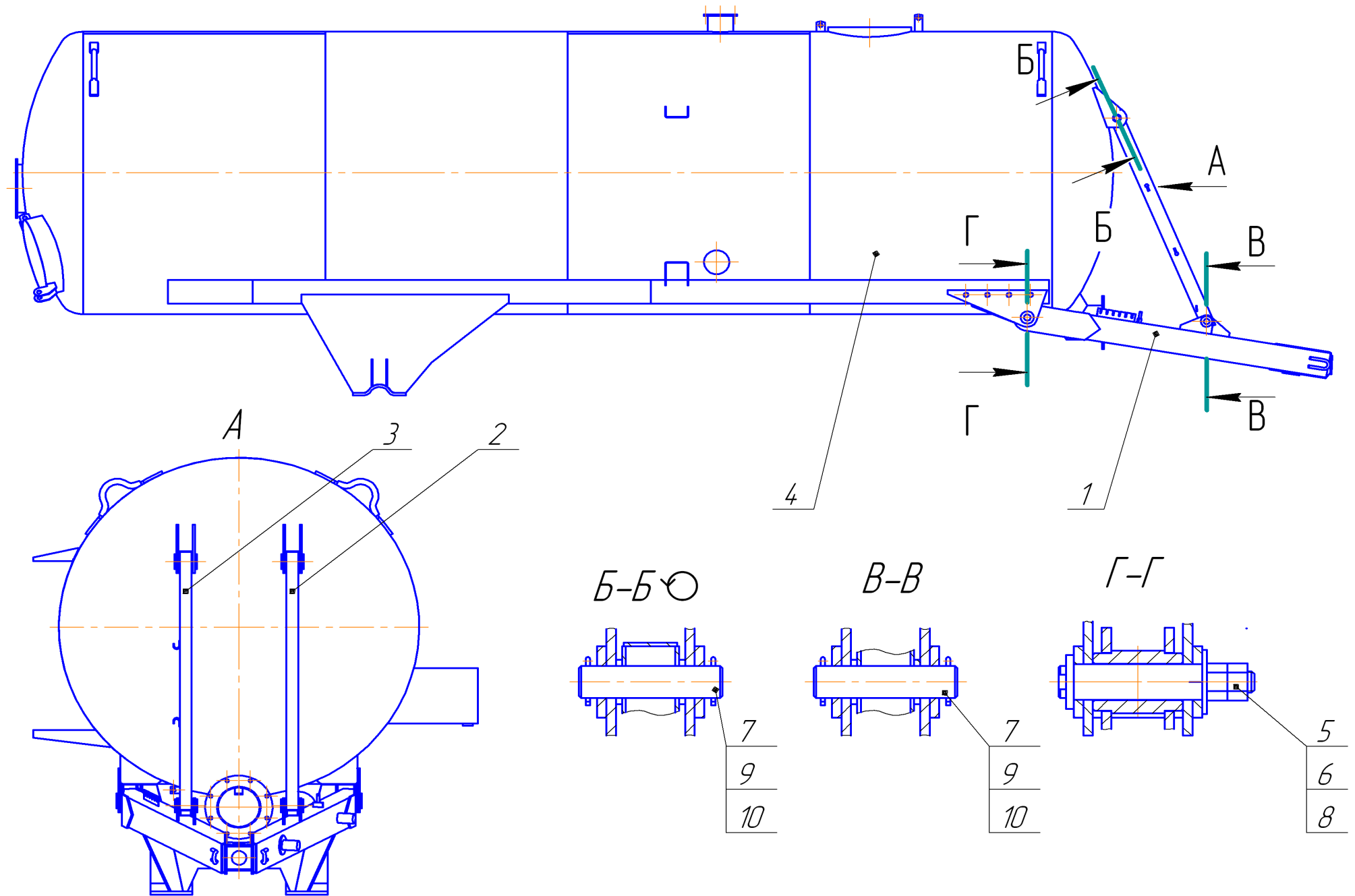
Рисунок 2 – Цистерна с дышлом МЖУ-16.42.00.000
